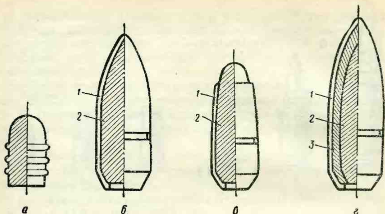
Рис. 7. Устройство пуль:
