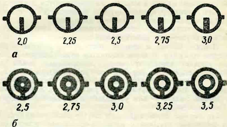
Рис. 5. Мушки:
