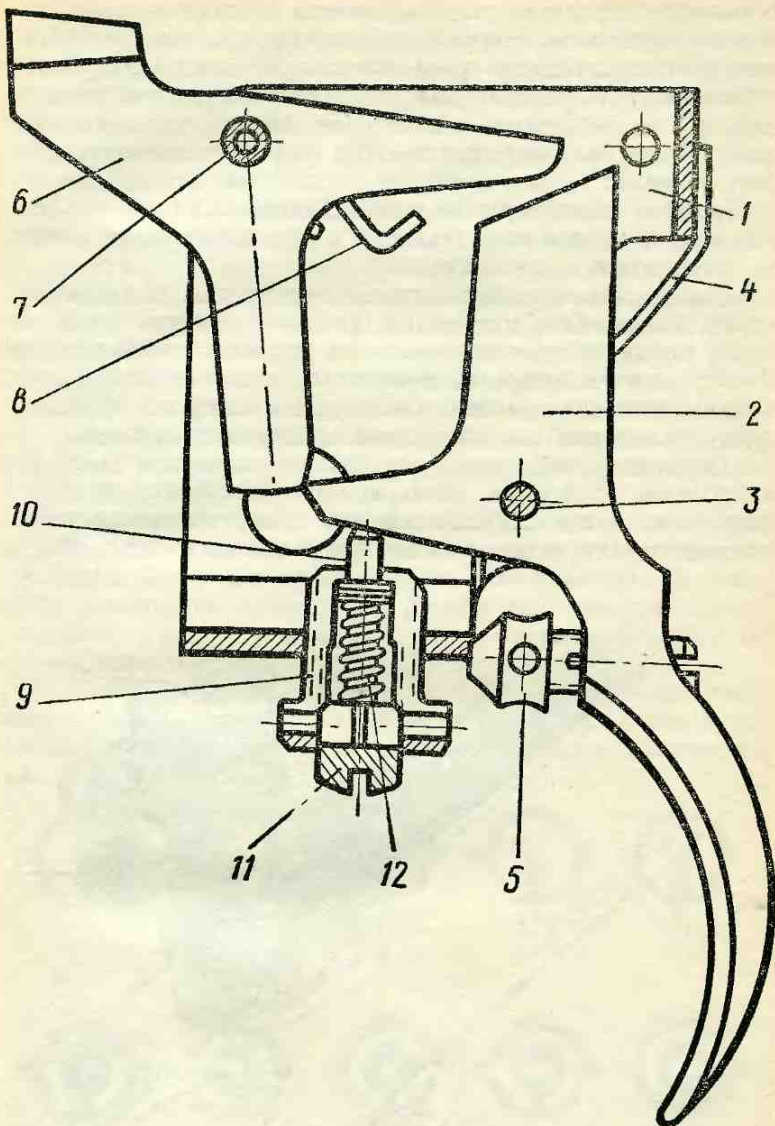
Рис. 3. Спусковой механизм:
