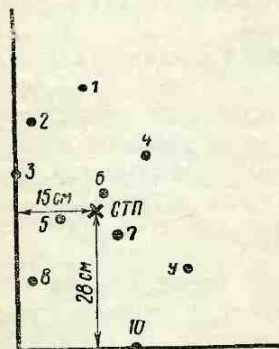
Рис. 2. Определение положения средней точки попадания способом вычисления (расчета).
