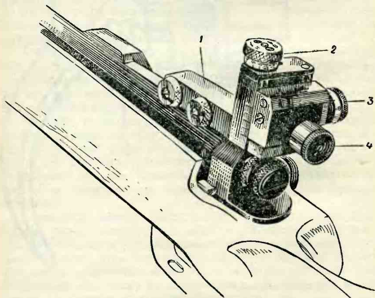
Рис. 4. Диоптрический прицел: 1 — основание прицела; 2 — головка винта вертикальных поправок; 3 — головка винта горизонтальных поправок; 4 — тарель с диоптром.
